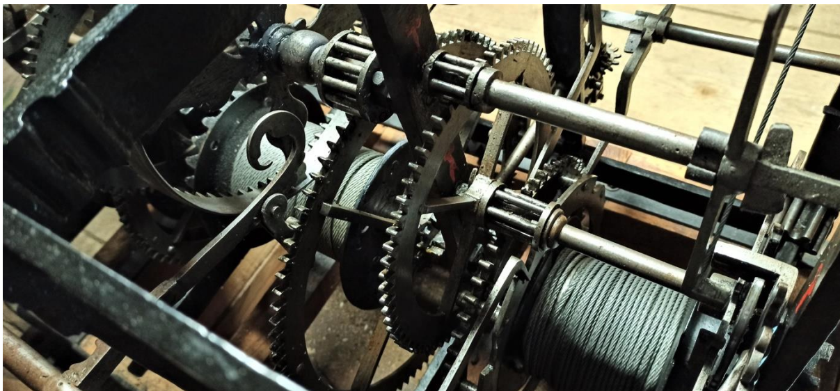
detail soukolí hodin
